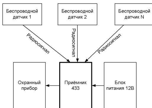
Рис.1 Принцип работы беспроводной системы охраны
