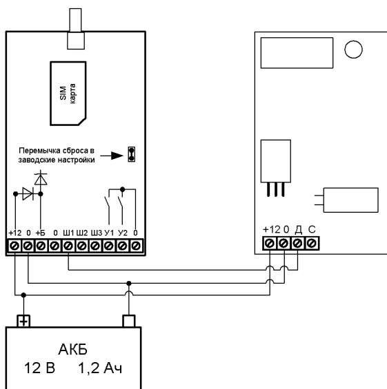
Рис. 2 Схема электрическая подключения приёмника 433 к охранному GSM-прибору SLX-3.
